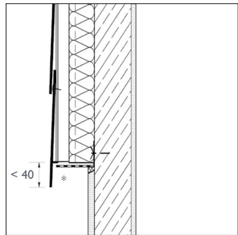
Sockel* (Vertikalschnitt)
