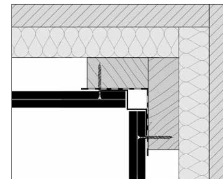
Innencke mit Inneneckprofil (Horizontalschnitt)
