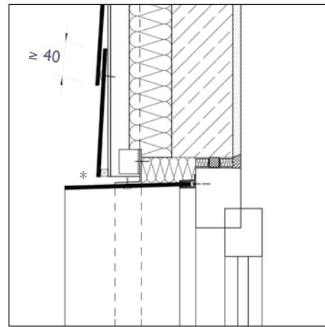
Fenstersturz* (Vertikalschnitt)
