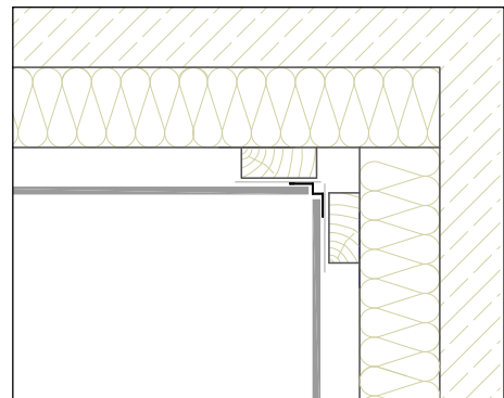
Innenecke mit Inneneckprofil (Horizontalschnitt)
