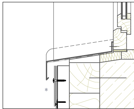
Fensterbrüstung* (Vertikalschnitt)
