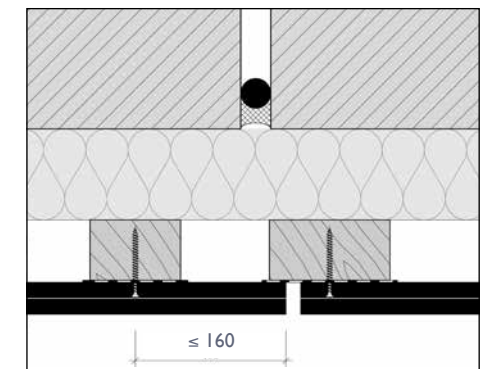
Dehnfuge (Horizontalschnitt)
