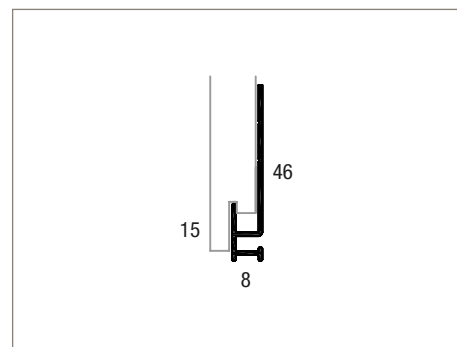
Cedral click Horizontal-Starterprofil (E)
