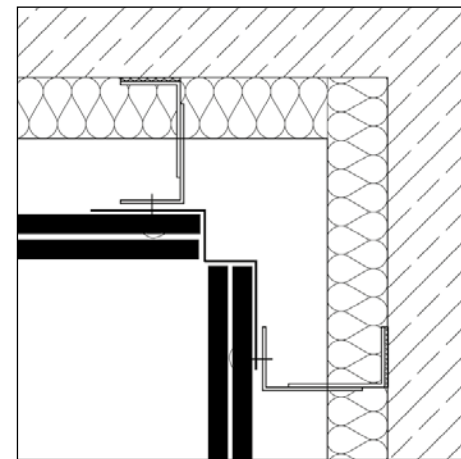
Innenecke mit Profil (Horizontalschnitt)
