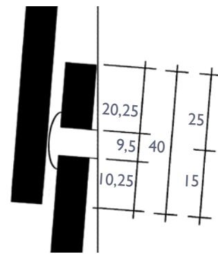
Vertikalschnitt – Abstände und Bohrung; Maße in mm
