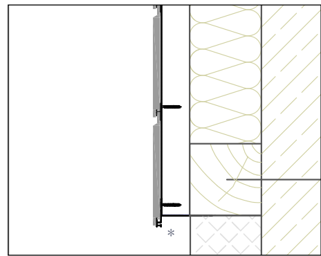
Sockelabschluss* (Vertikalschnitt) mit Starterprofil
