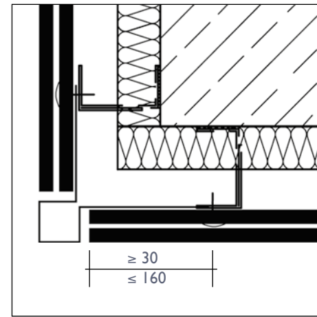
Außenecke mit Profil (Horizontalschnitt)
