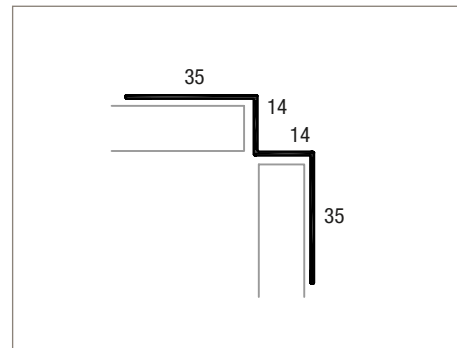
Cedral click Inneneckprofil (B)
