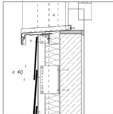
Fensterbrüstung* (Vertikalschnitt)
