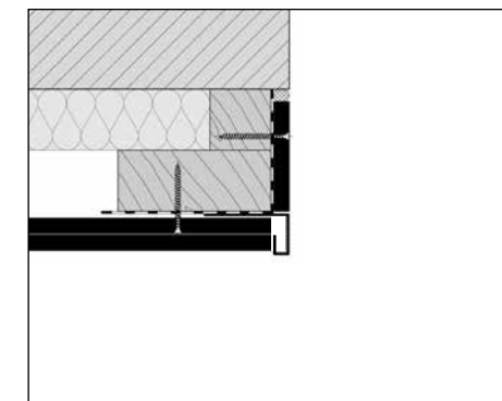
Seitlicher Abschluss mit Abschlussprofil (Horizontalschnitt)
