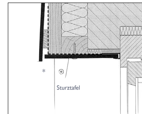
Fenstersturz* (Vertikalschnitt)
