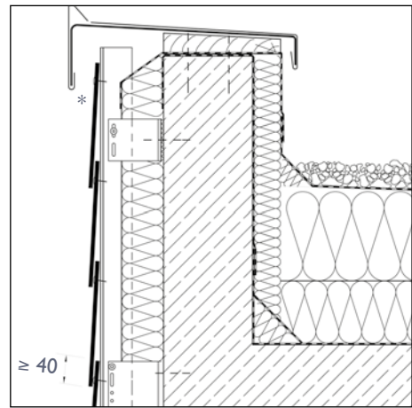
Attika* (Vertikalschnitt)
