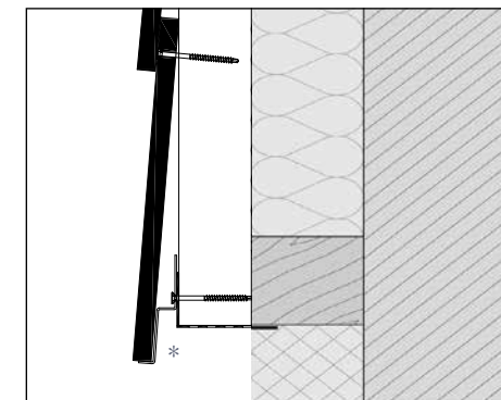
Sockelabschluss* (Vertikalschnitt)
