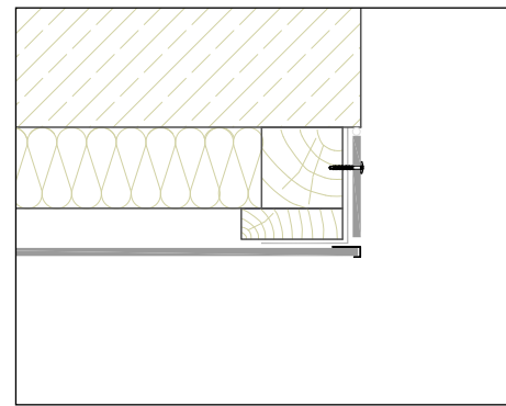
Seitlicher Abschluss mit Cedral Fensteranschlussprofil (Horizontalschnitt)
