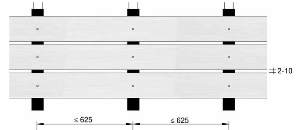
Horizontal verlegte Cedral Lap Fassadenpaneele auf vertikaler Traglattung (Windzone I + II bis 10 m Gebäudehöhe); Maße in mm.
