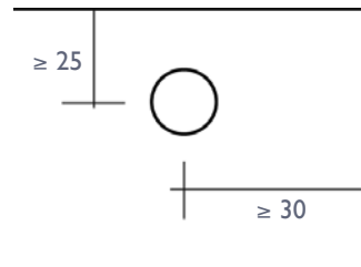
Einzuhaltende Mindestrandabstände der Bohrung \varnothing 9,5 mm von der Paneelkante
