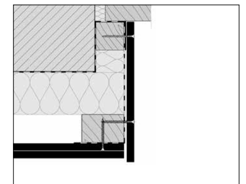
Fensterleibung ohne Leibungsprofil (Horizontalschnitt)
