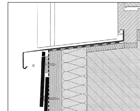
Fensterbrüstung* (Vertikalschnitt)
