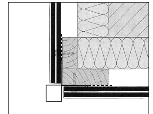
Außencke mit Eckprofil (Horizontalschnitt)
