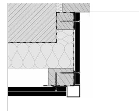
Fensterleibung mit Leibungsprofil
