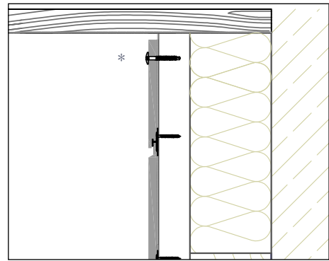
Anschluss am Dachüberstand mit sichtbarer Fassadenschraube am oberen Rand* (Vertikalschnitt)
