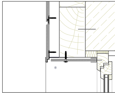
Fenstersturz (Vertikalschnitt) mit Sturzprofil*
