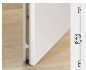
Dreifachverriegelung, Bodendichtung und Türaufschlagdichtung
